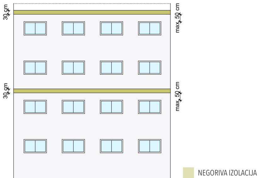
Slika 33 Sprečavanje vertikalnog širenja požara pomoću horizontalnog kontinuiranog pojasa od negorivog materijala ugrađenog na pročelju svake druge etaže [15]
