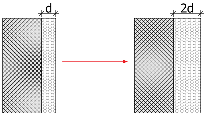
Slika 5 Povećanje debljine toplinskoizolacijskog sloja zbog energetske učinkovitosti zgrada
