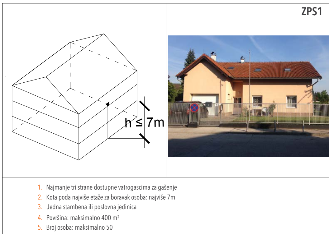
Slika 18 Shematski prikaz tipične zgrade podskupine 1 s fotografijom
