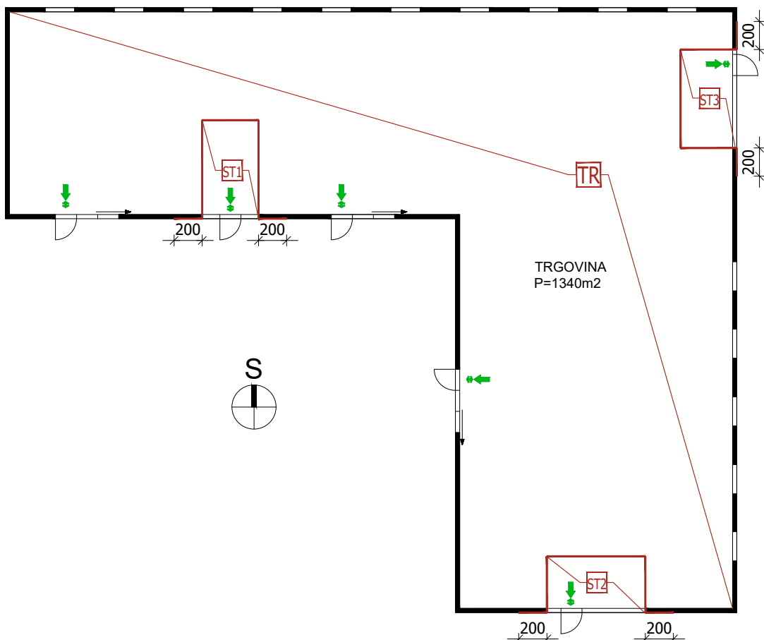
Slika 46 Shematski prikaz prizemlja - tlocrt
